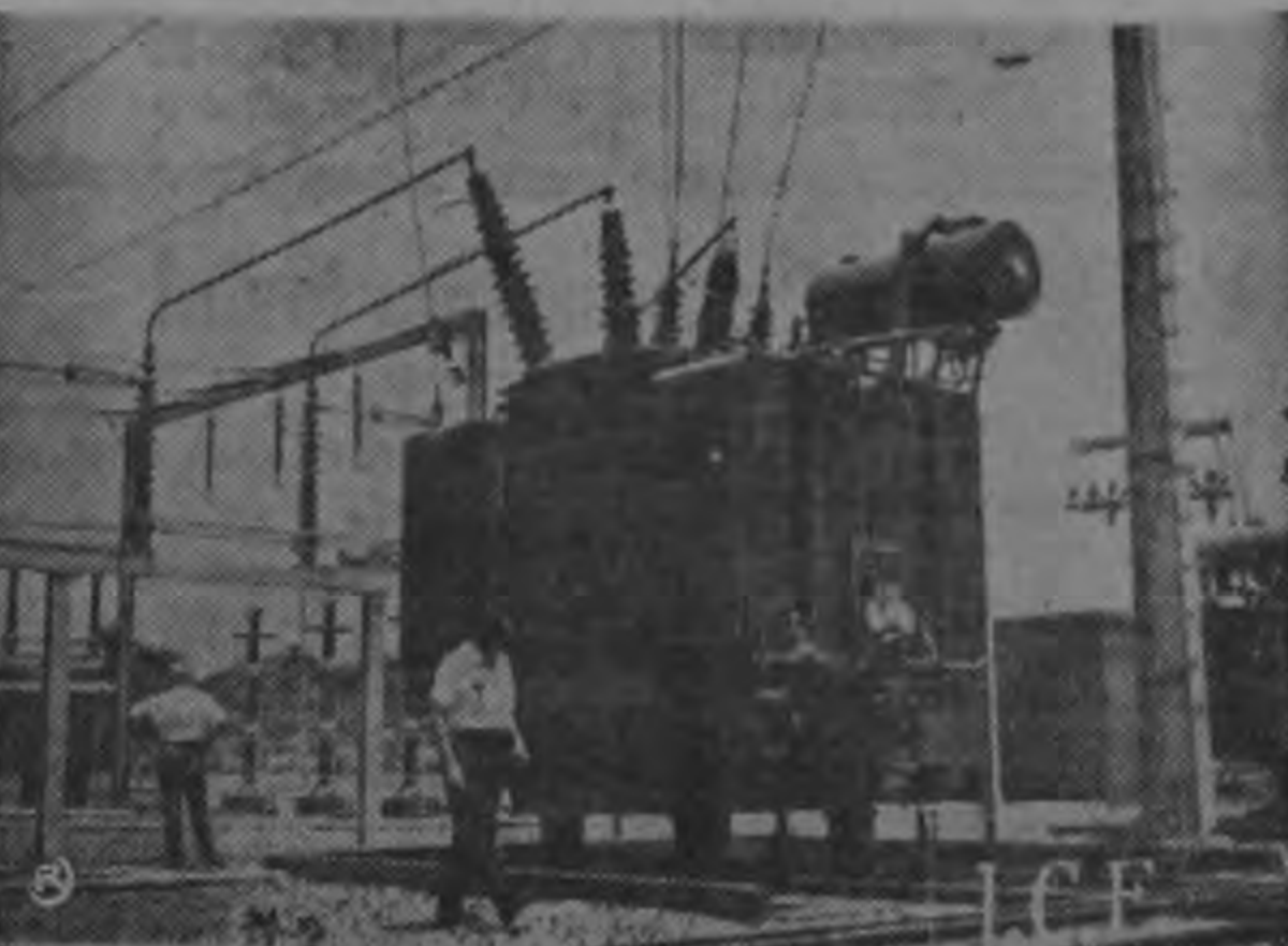
ENORMES TRANSFORMADORES instalados en el patio de la sub-estación del ICE en Barranca, garantizan una entrega de energía eléctrica constante y un servicio de la mejor calidad. Las inversiones del ICE en el área del Pacífico han sido considerables.
